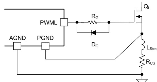
図 7-15. Driving a Si MOSFET
