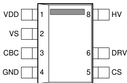
図 4-1. D Package 7-Pin SOIC Top View
