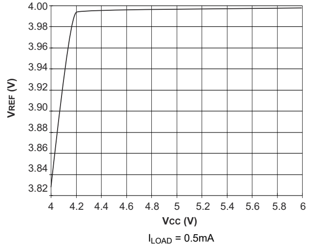
図 6-2. UCC3813-[3, 5]: V_{\text{REF}} と V_{\text{CC}} との関係
