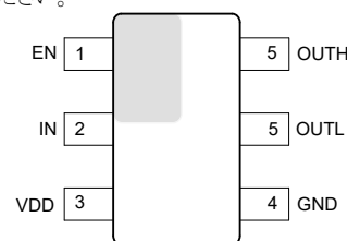
ピン配置
