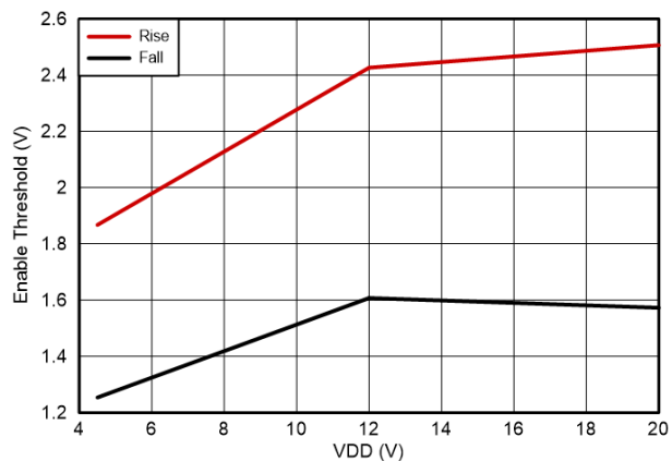
FIG 6-8. Enable Threshold
