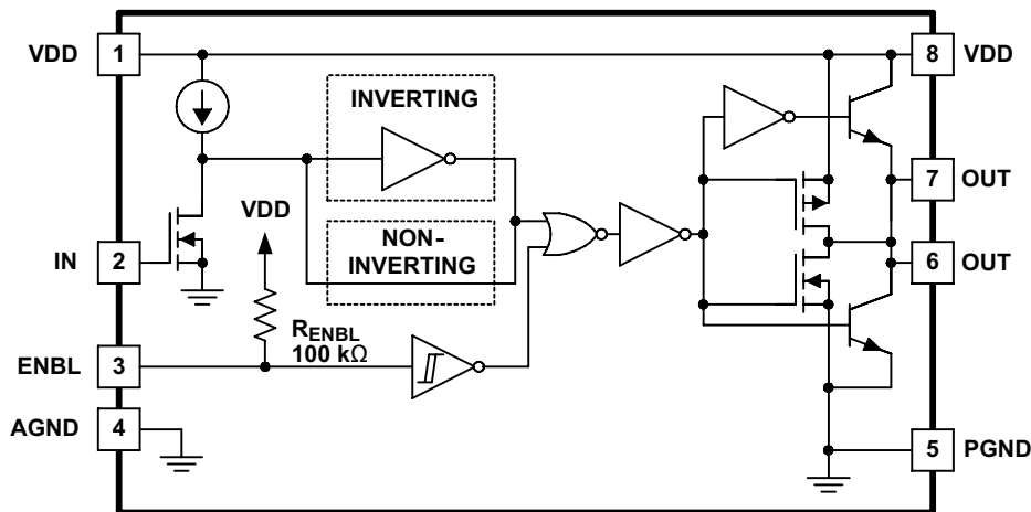
ブロック図
