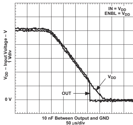
図 9-3. Output Behavior vs VDD (UCC37322)
