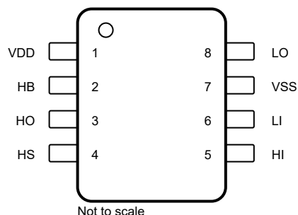
図 4-1. D パッケージ 8 ピン SOIC 上面図
