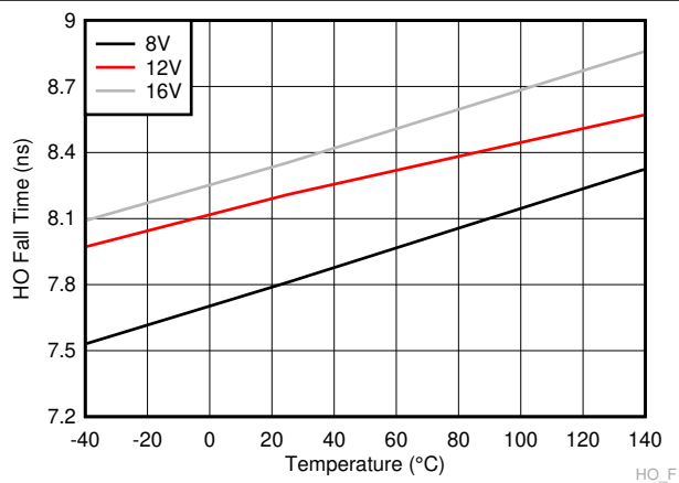
6-19. HO Fall Time
