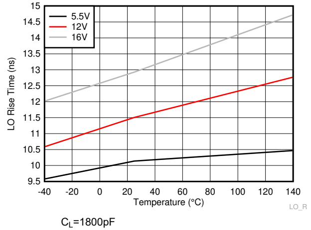
6-22. LO Rise Time
