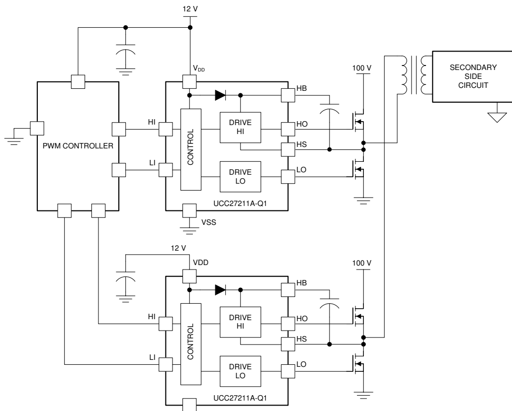
図 7-2. UCC27211A-Q1 代表的なアプリケーション図 2
