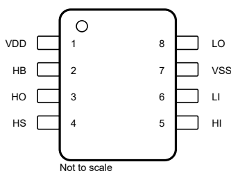
図 4-2. D パッケージ 8 ピン SOIC 低面図
