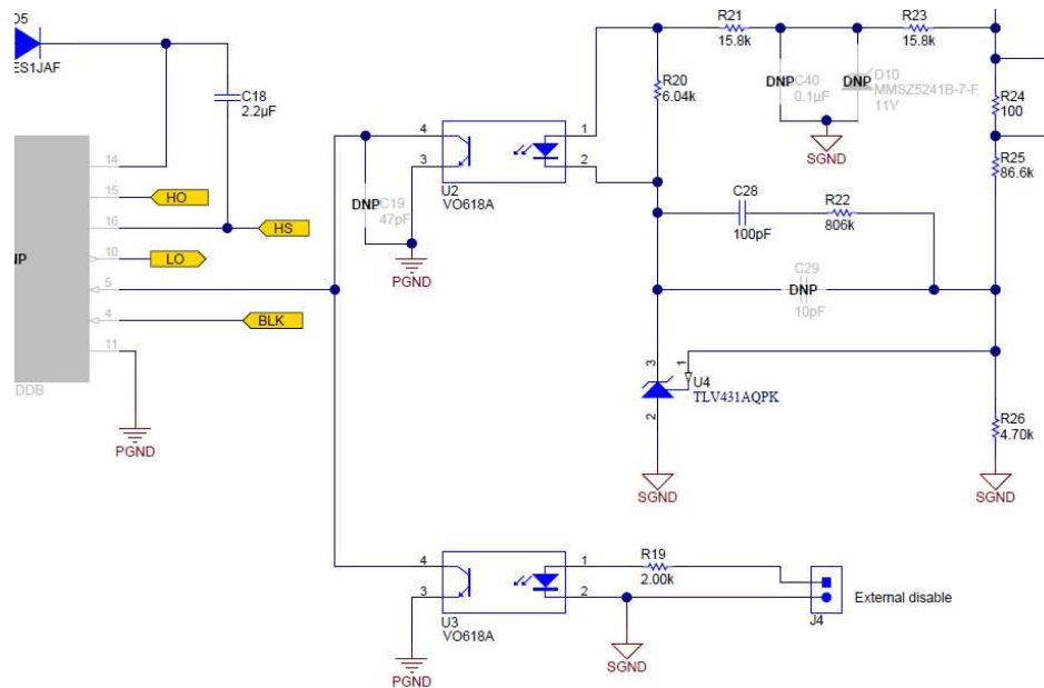
図 32. 外部ディセーブル回路例
