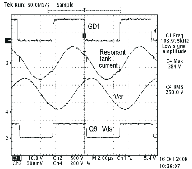
図 8-13. 標準的な共振タンク電流と共振コンデンサ電圧
