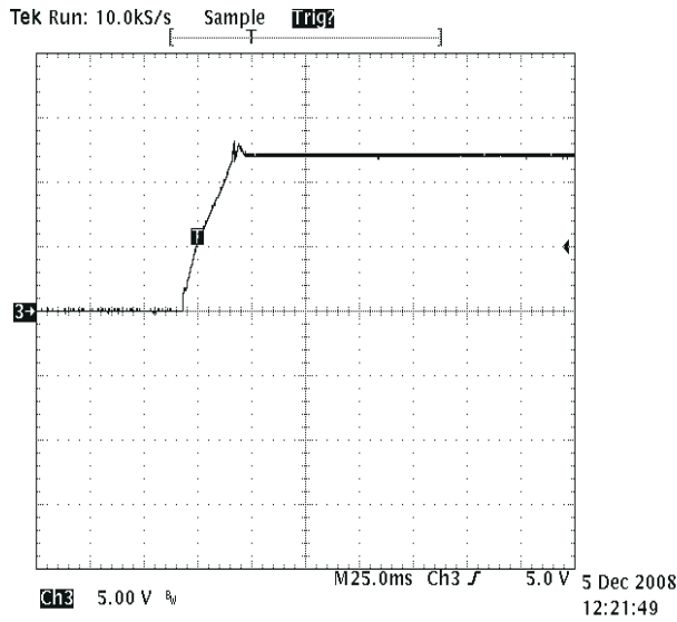
図 8-10. 標準的な出力電圧ターン オン (TP15)
