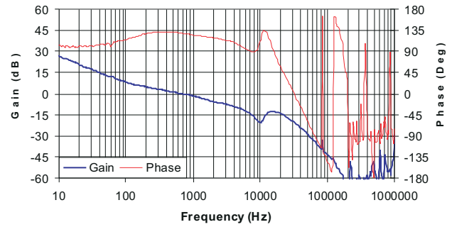
図 8-11. 完全なシステム ループ補償 (TP19 および TP21)
