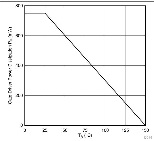
図 6-2. VDE に従う制限電力の熱特性低下曲線
