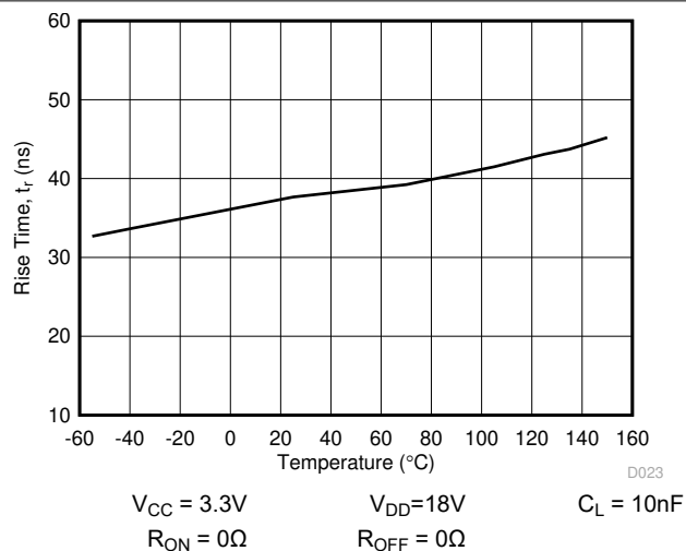
图 5-15. t_r Rise Time vs Temperature
