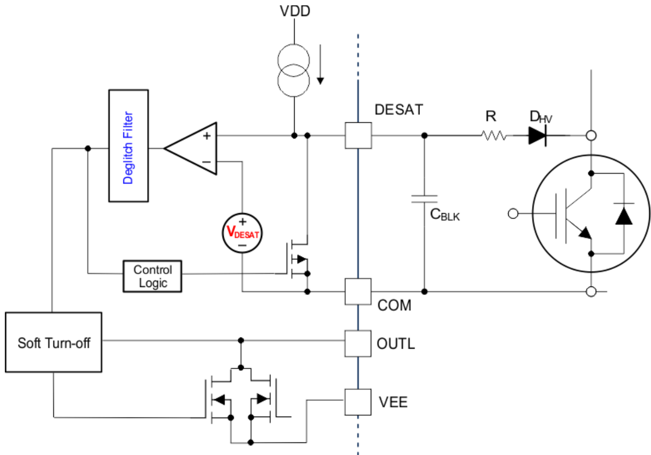
図 8-6. Soft Turn-Off
