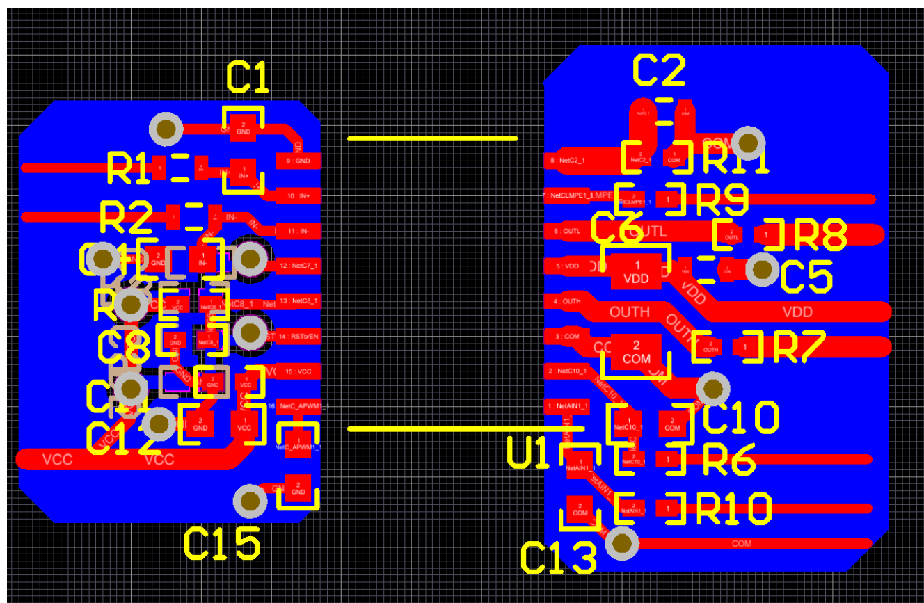
図 11-1. Layout Example
