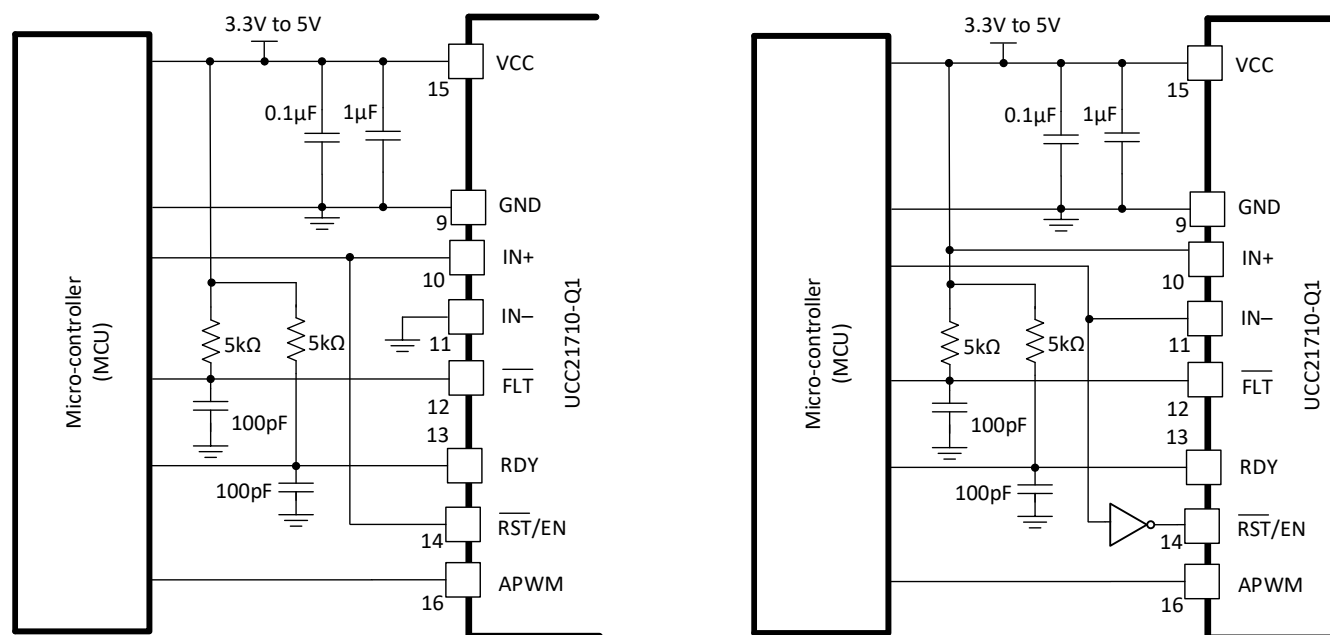
図 8-4. Automatic Reset Control
