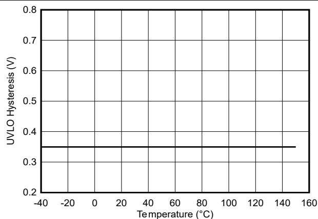
図 5-20. VDD 5V UVLO ヒステリシスと温度との関係
