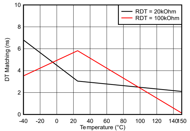
図 5-31. デッド タイム マッチングと温度との関係 ( R_{DT} = 20\text{k}\Omega および 100\text{k}\Omega の場合)
