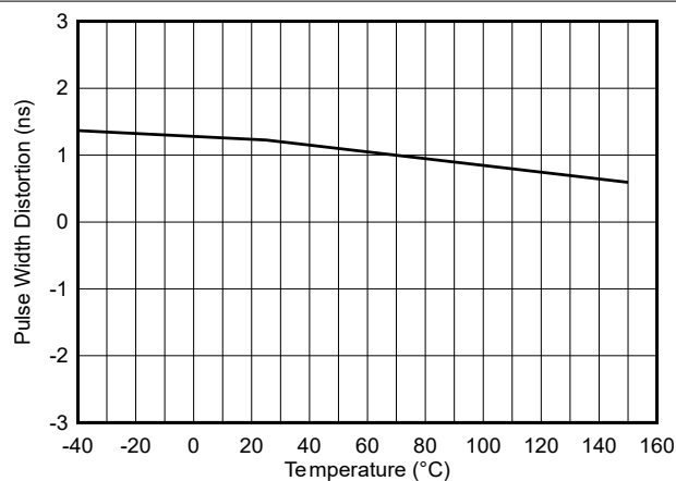
図 5-16. パルス幅歪みと温度との関係
