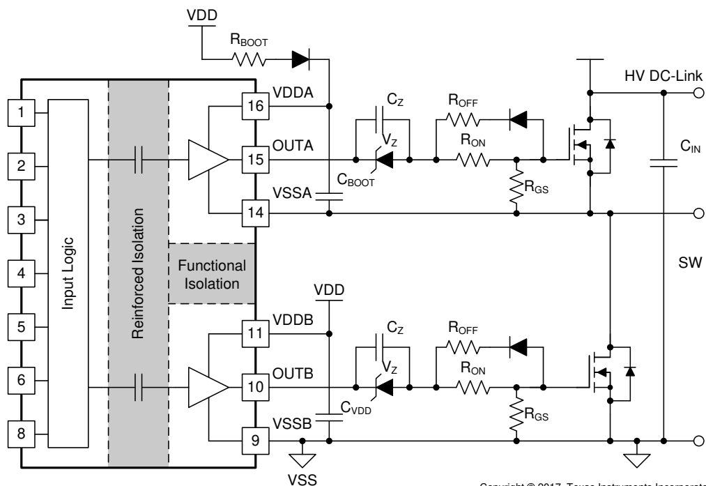
図 8-4. 1 つの電源とゲート駆動経路内のツェナー ダイオードによる負バイアス印加
