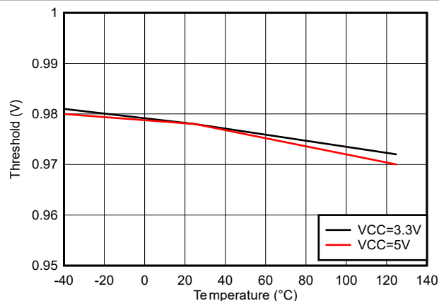
図 5-28. IN/EN の Low スレッシュホールド
