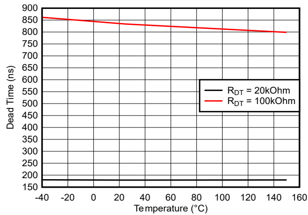
図 5-30. デッド タイムと温度との関係 ( R_{DT} = 20\text{k}\Omega および 100\text{k}\Omega の場合)
