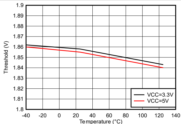
図 5-29. IN/EN の High スレッシュホールド
