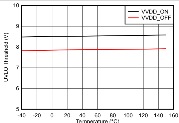
図 5-21. VDD 8V UVLO スレッシュホールドと温度との関係
