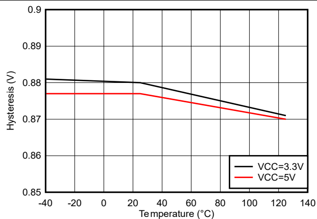
図 5-27. IN/EN ヒステリシスと温度との関係
