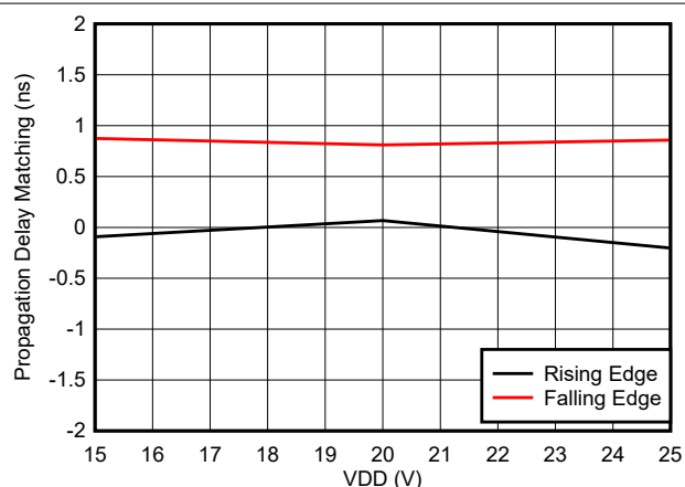
図 5-17. 伝搬遅延マッチング ( t_{\text{DM}} ) と VDD との関係
