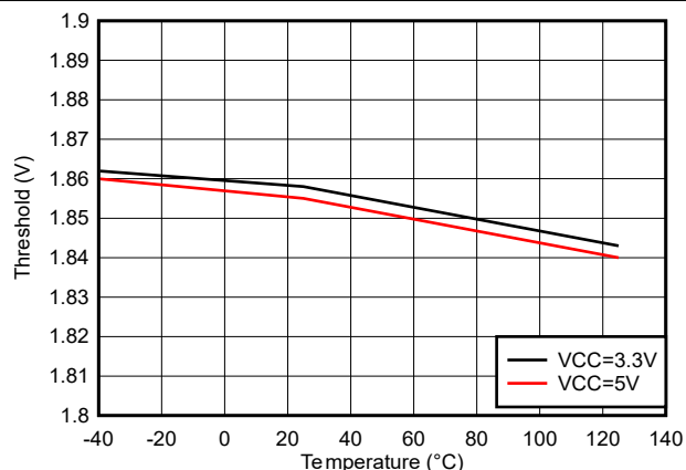
図 5-25. IN/DIS の High スレッシュホルド
