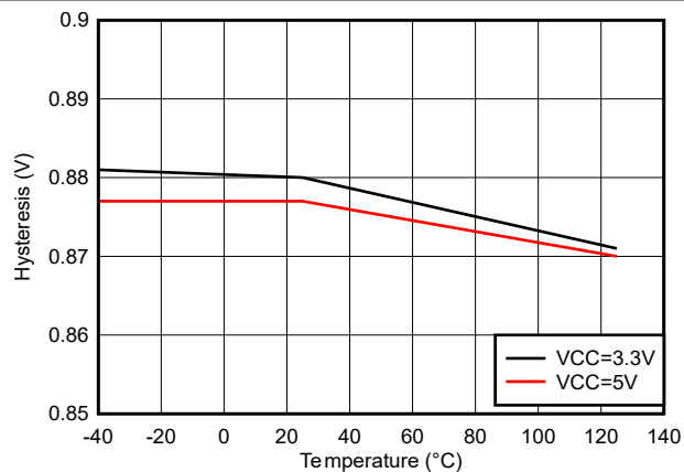
図 5-23. IN/DIS ヒステリシスと温度との関係
