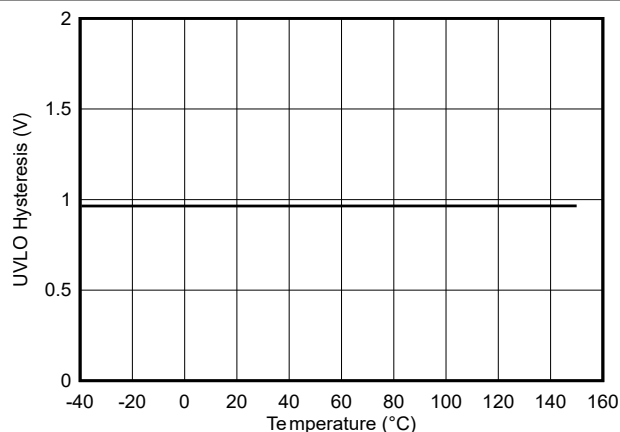
図 5-22. VDD 12V UVLO ヒステリシスと温度との関係
