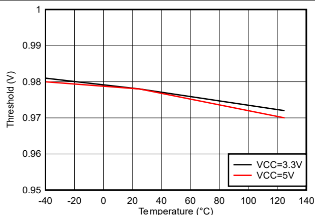
図 5-24. IN/DIS の Low スレッシュホルド
