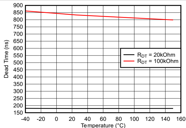
図 5-26. デッド タイムと温度との関係 ( R_{DT} = 20\text{k}\Omega および 100\text{k}\Omega の場合)
