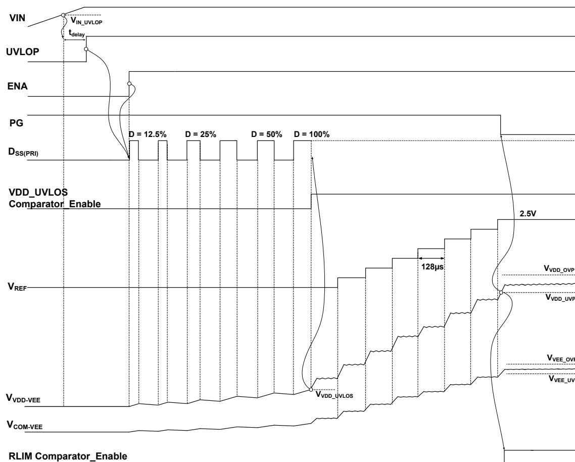
图 11-5. Output voltage Soft-Start Diagram
