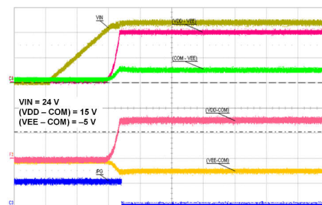
代表的な電源投入シーケンス
