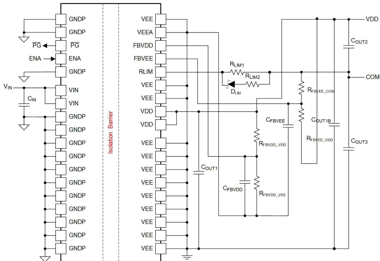
图 8-10. 双输出应用电路示意图，配置为 V_{COM\_VEE} 调节 < 2.5V
