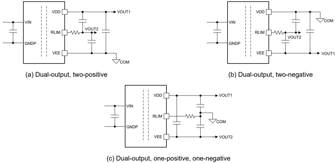
図 8-6. Dual output configurations
