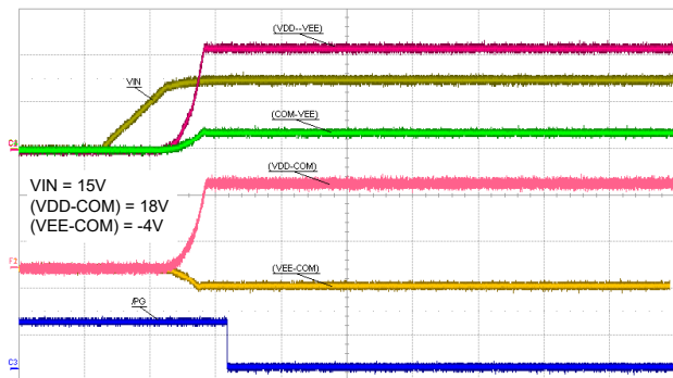
代表的な電源投入シーケンス
