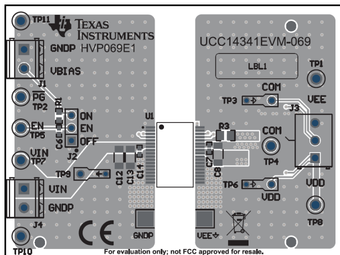
図 12-9. UCC14340-Q1EVM, PCB Top Layer, Assembly
