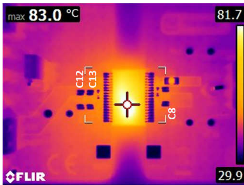
图 9-15. Thermal Image
