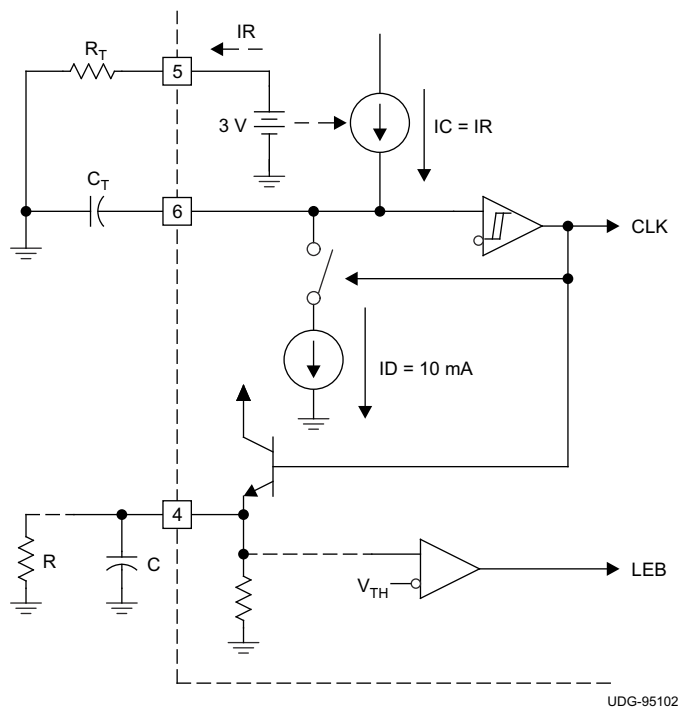
図 8-1. Oscillator
