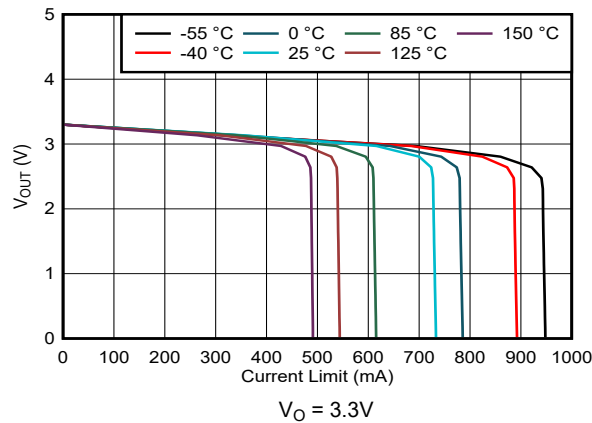
図 5-7. Output Voltage vs I_{CL} (New Chip)
