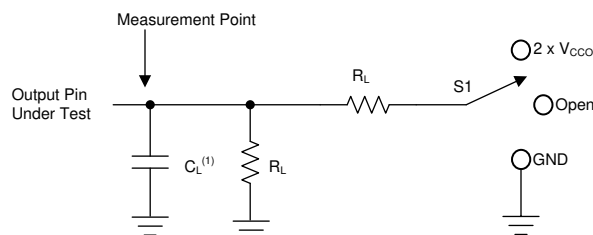
図 6-1. 負荷回路
