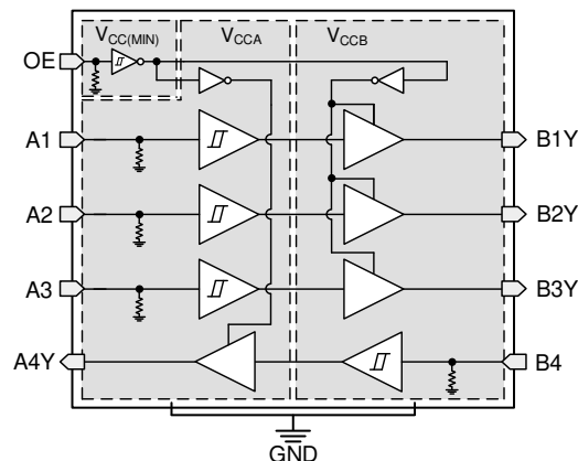
TXU0304 機能ブロック図
