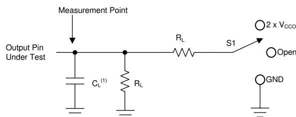
图 6-1. Load Circuit
