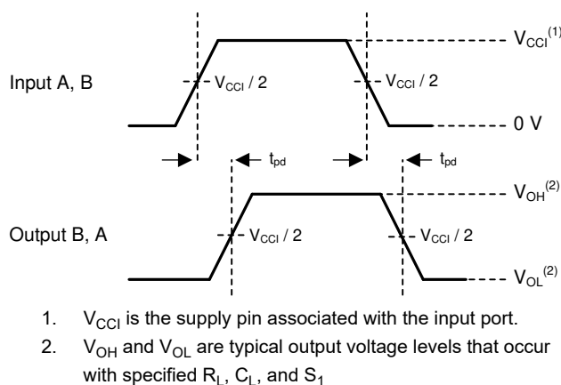
图 6-2. Propagation Delay
