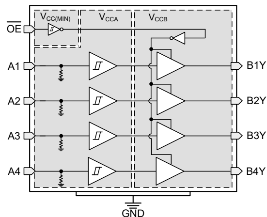
TXUN0104 の機能ブロック図
