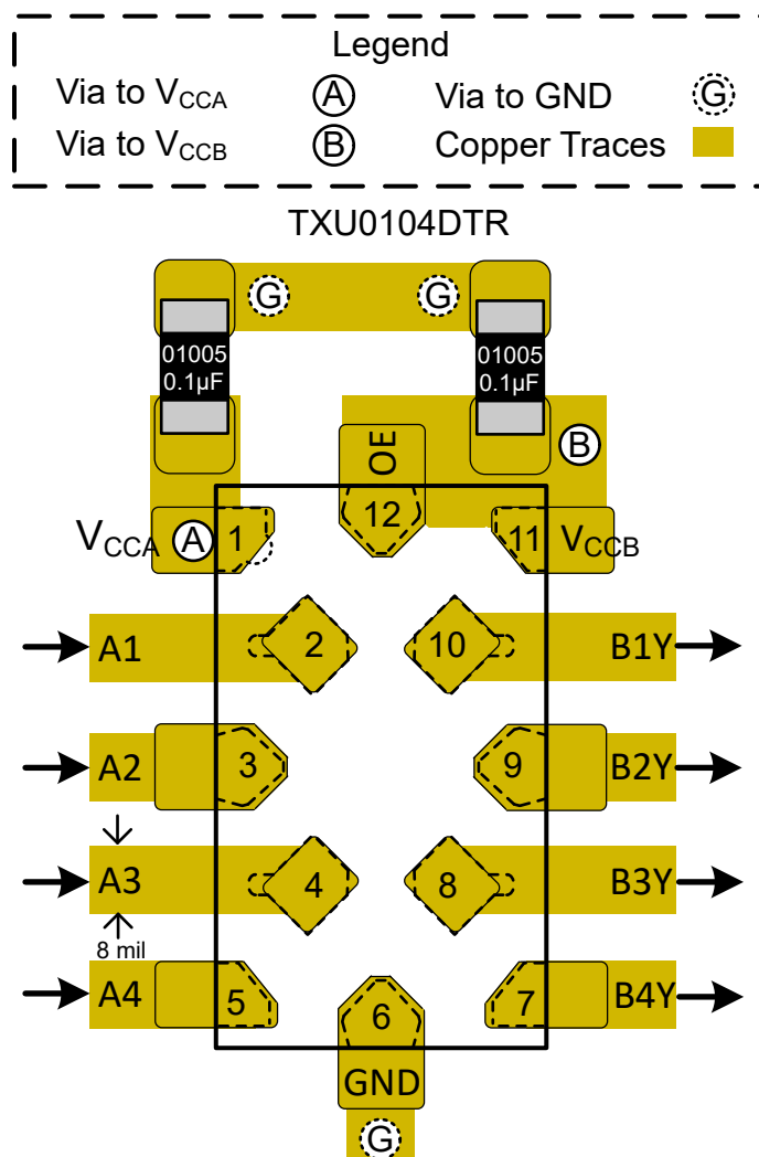
図 8-3. Layout Example – TXU0104
