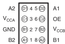
図 4-1. YZP パッケージ、8 ピン DSBGA (底面図)
