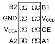
図 4-4. DTT パッケージ、8 ピン SOP (上面図)
