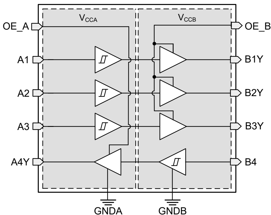
TXG8041-EP の機能ブロック図
