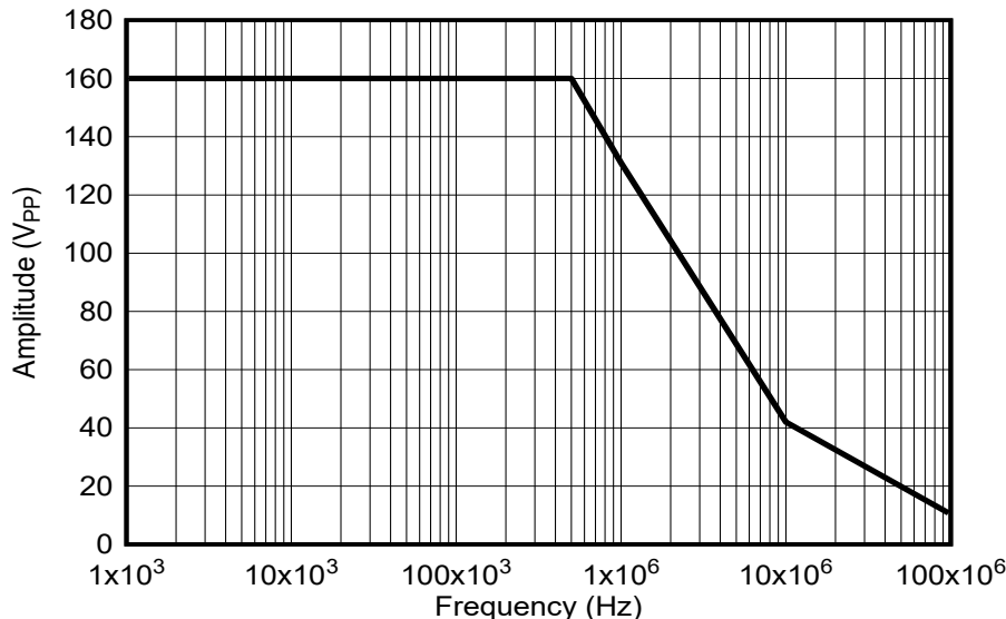
図 7-3. AC ノイズ除去プロット
