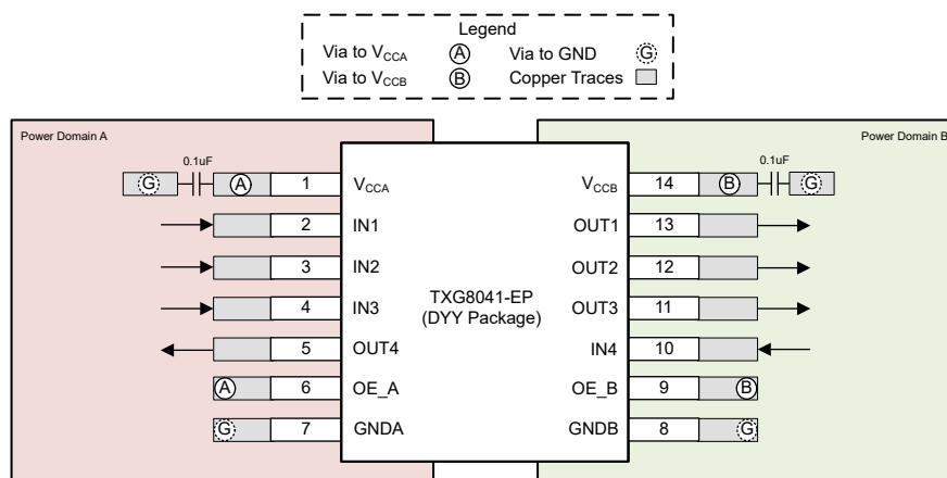
図 8-3. DYY のレイアウト例
