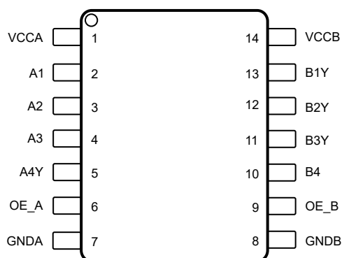
図 4-1. TXG8041-EP DYY 14 ピン SOT 上面図
