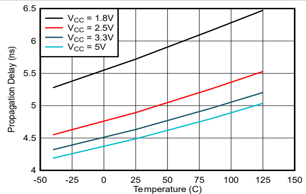
図 5-6. 伝搬遅延、 T_{PHL} 、と温度との関係
