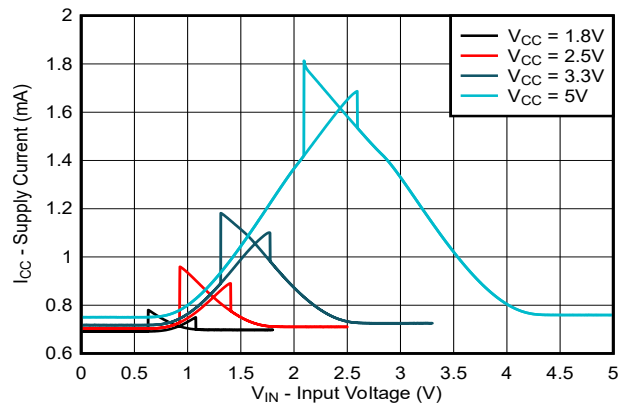
図 5-3. 電源電流 ( I_{CC} ) と入力電圧 ( V_{IN} ) との関係 [TXG0x041]
