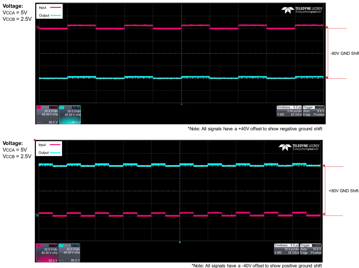
図 8-2. 5V から 2.5V への I/O 変換による -80V (上) および +80V (下) のグラウンド シフトを示す波形
