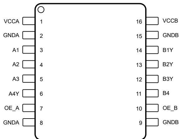
図 4-3. TXGx041 DBQ 16 ピン QSOP 上面図
