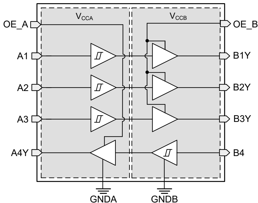
TXG804x の機能ブロック図
