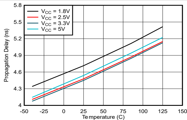
図 5-5. 伝搬遅延、 T_{PLH} 、と温度との関係
