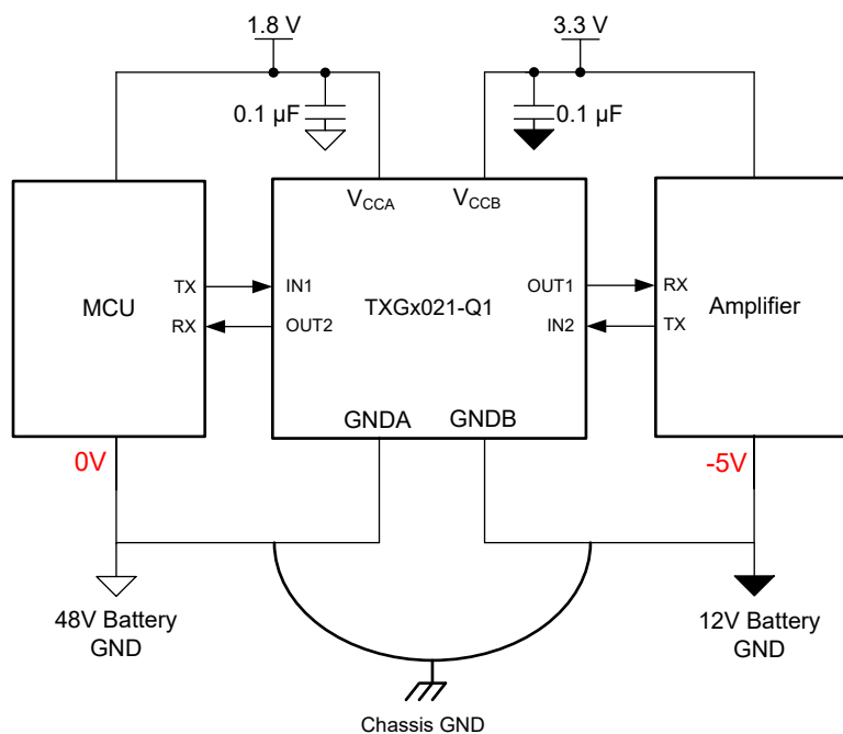
図 8-1. 車載用途での TXG8021-Q1
