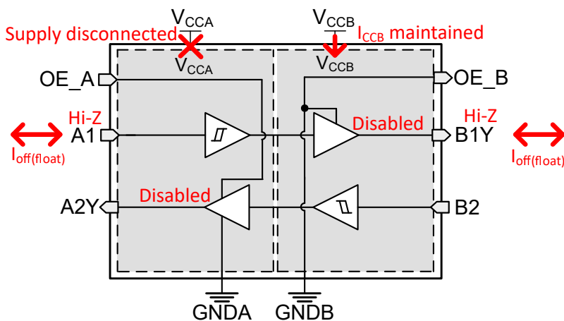
図 7-2. V CC 接続解除機能
