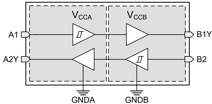
図 7-1. TXG8021-Q1 機能ブロック図
