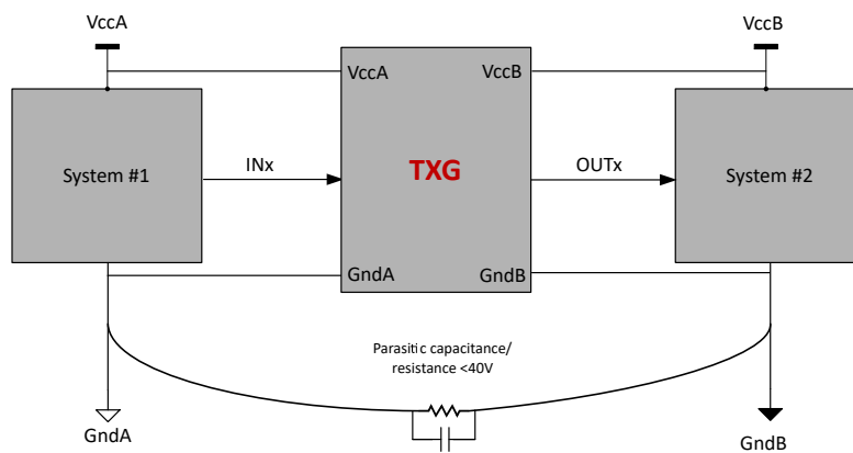
簡略ブロック図
