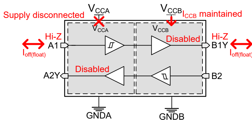
図 7-2. V_{CC} 接続解除機能
