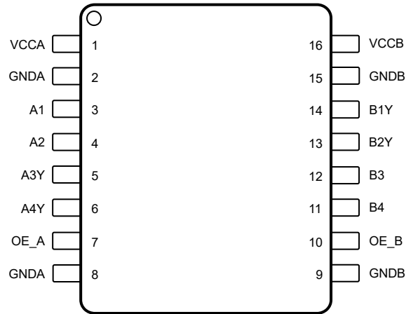
図 4-6. TXG1042-Q1 DBQ 16 ピン QSOP 上面図
