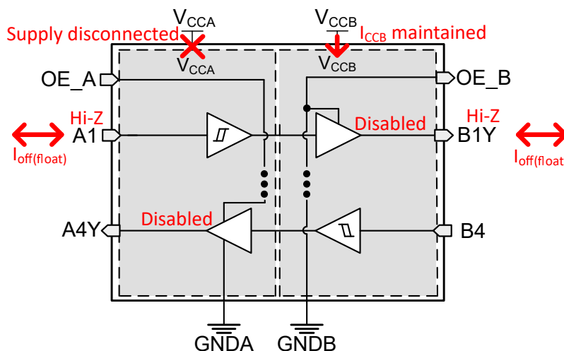
図 7-2. V CC 接続解除機能
