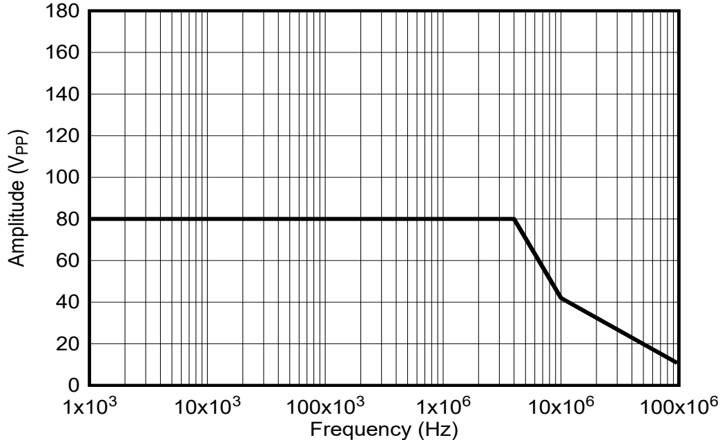
図 7-4. AC ノイズ除去プロット
