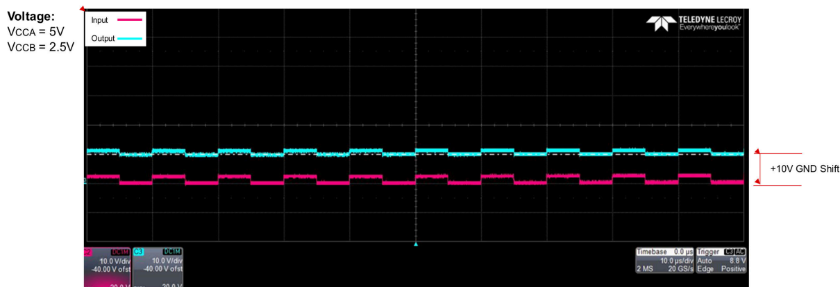
図 8-2. 5V から 2.5V への I/O 変換による -10V（上）および+10V（下）のグラウンド シフトを示す波形
