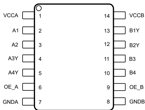
図 4-4. TXGx042DYY 14 ピン SOT 上メンズ
