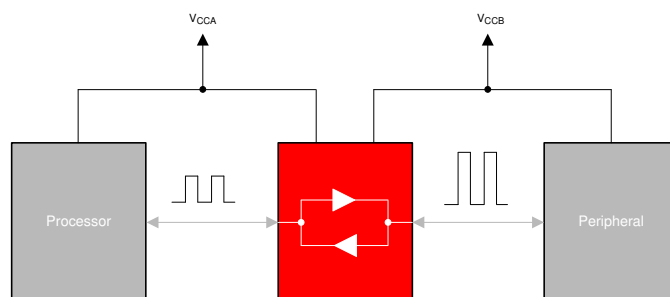
TXB0108-Q1 の代表的なアプリケーション ブロック図
