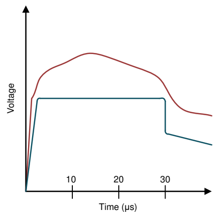
8μs~20μs のサージに対する電圧クランプの応答
