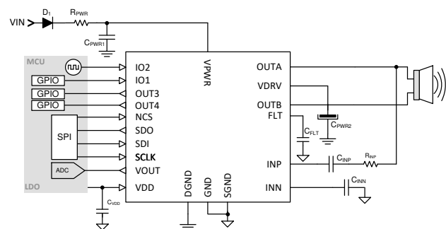
TUSS4470 アプリケーション図
