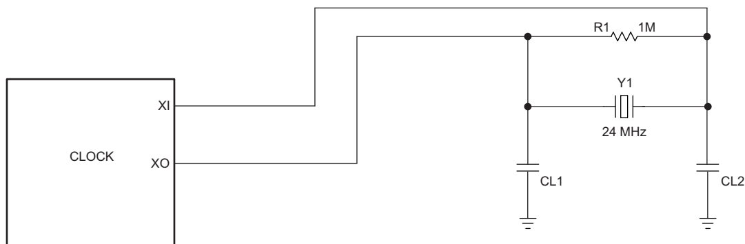
图 2. TUSB8044A Clock
