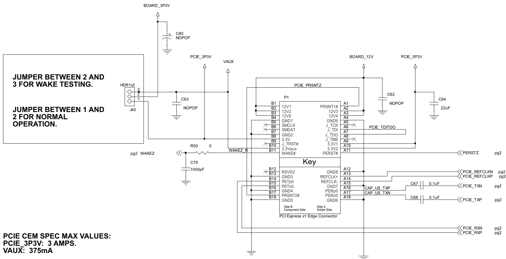
図 7-5. Reference Design 3
