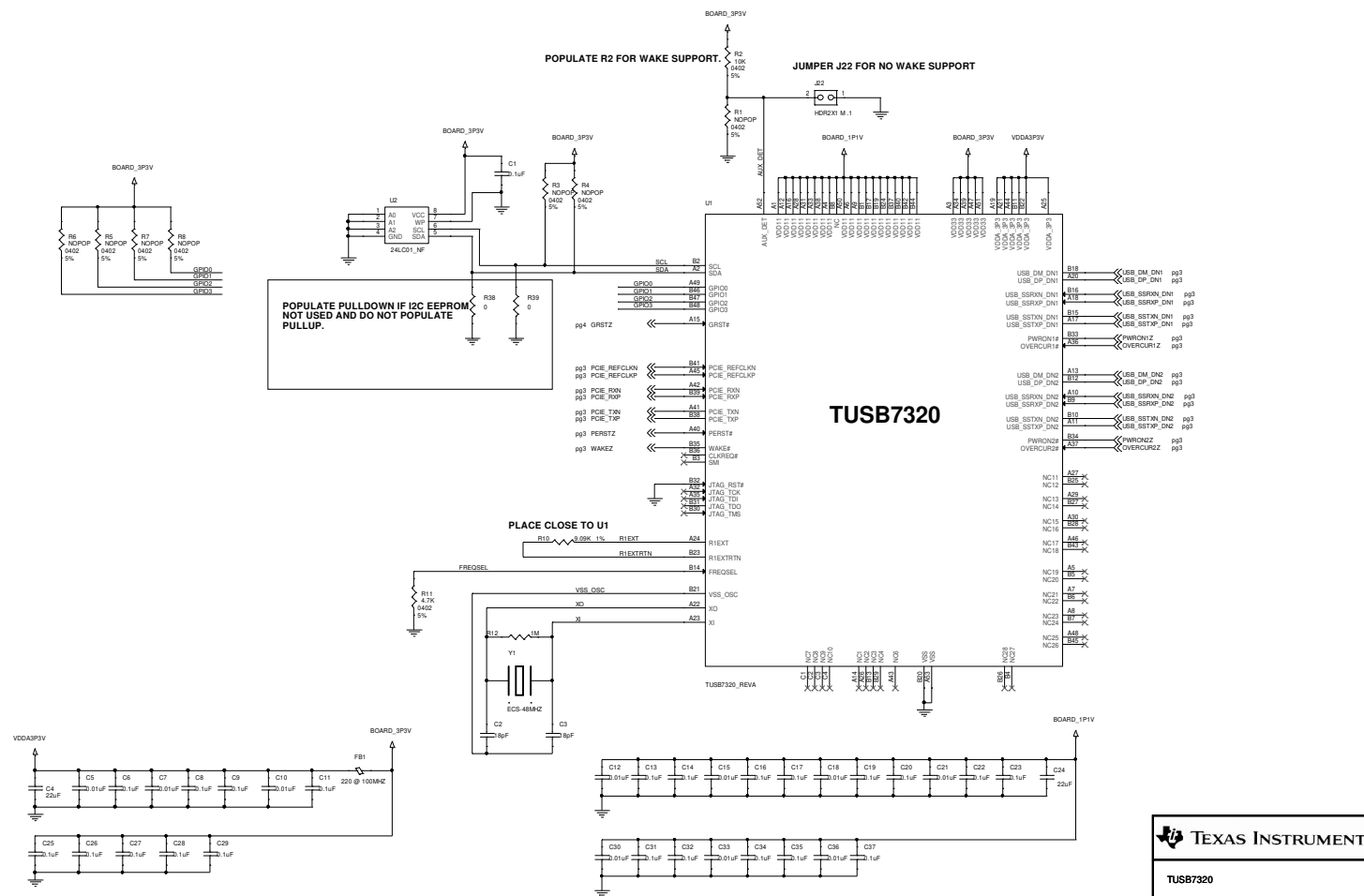
图 7-3. Reference Design 1
