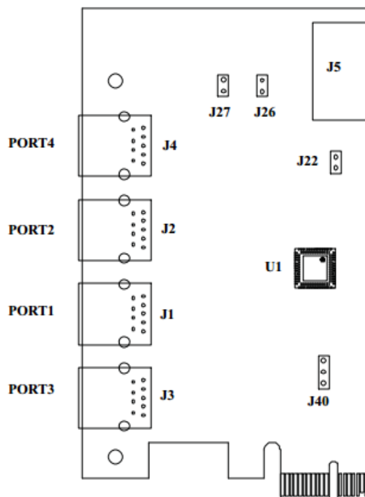
図 7-2. TUSB7340 DEMO EVM REV B
