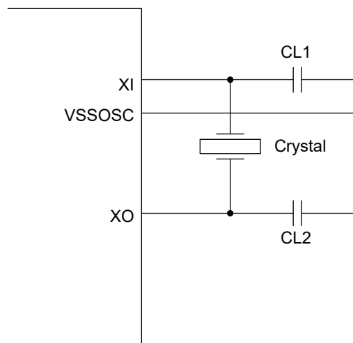
図 6-1. Oscillation Circuit
