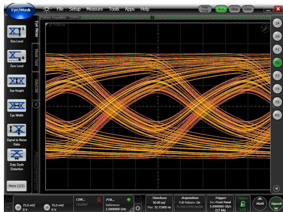
図 5-7. Input Signal: 24-Inch Input Trace
