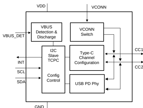
概略回路図
