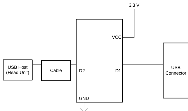
概略回路図
