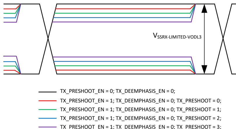
図 6-9. SSRX 制限プリシュートのみ
