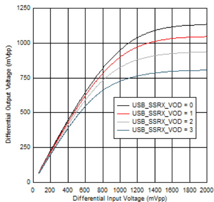
図 5-19. 5GHz での USB SSRX VOD 直線性設定
