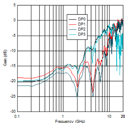
図 5-13. DisplayPort 出力のリターン ロス性能
