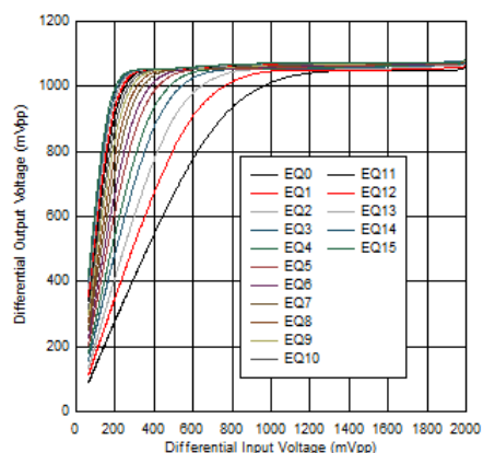
図 5-7. 4.05GHz での DisplayPort 直線性曲線
