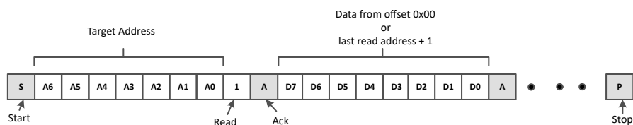
図 6-3. リピート スタートなしでの I 2 C 読み出し
