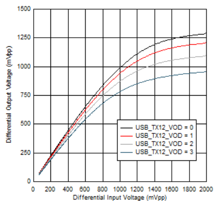
図 5-21. 5GHz での USB TX1 VOD 直線性設定
