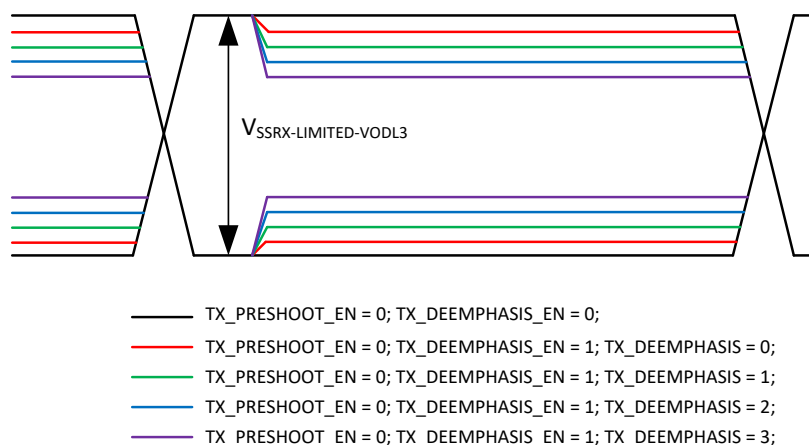
図 6-8. SSRX 制限ディエンファシスのみ
