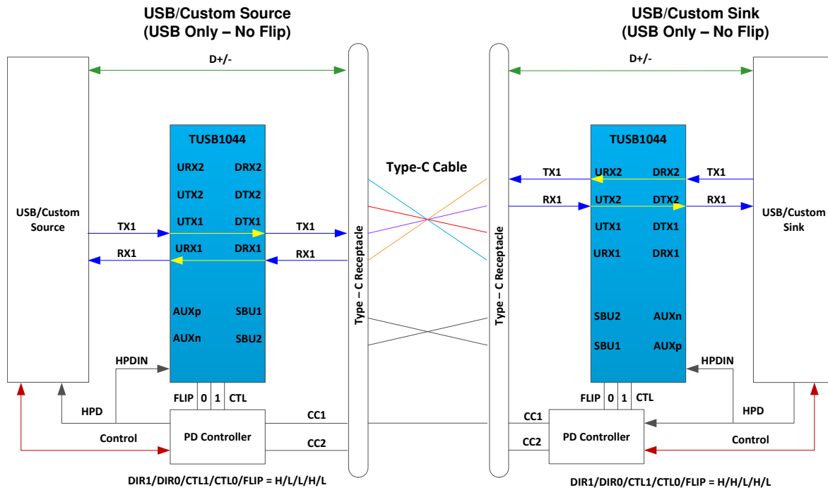
図 7-10. USB3.1 Only – No Flip
