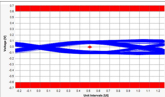
✎ 7-8. PCIe Gen3 TX Eye Diagram
