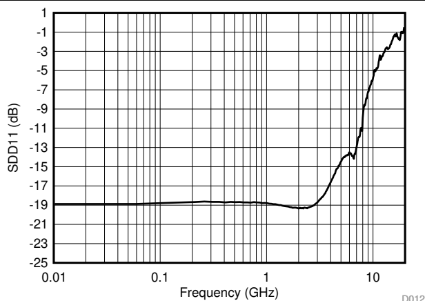
図 5-12. SDD11 Return Loss
