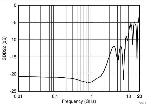
図 5-13. SDD22 Return Loss
