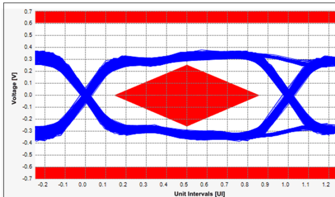
✎ 7-7. PCIe Gen1 TX Eye Diagram
