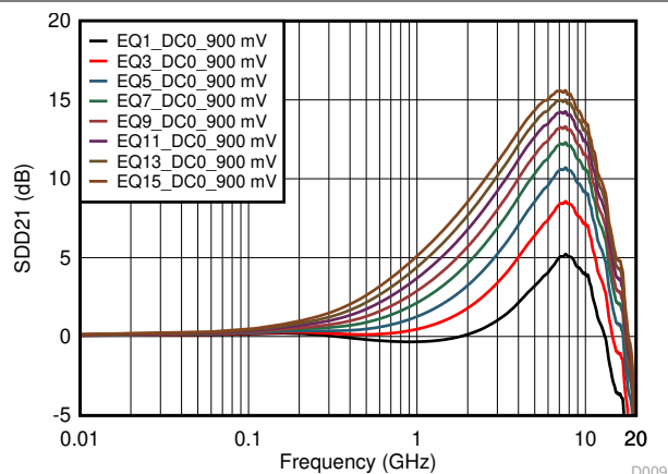
図 5-9. 900mV DC0 Gain Odd EQ Settings Curves
