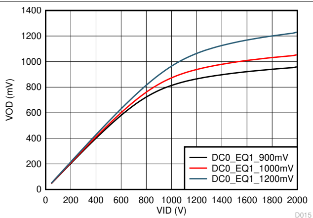
図 5-15. 100MHz Sine Wave VID vs VOD Linearity Range Setting
