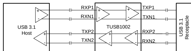
概略回路図
